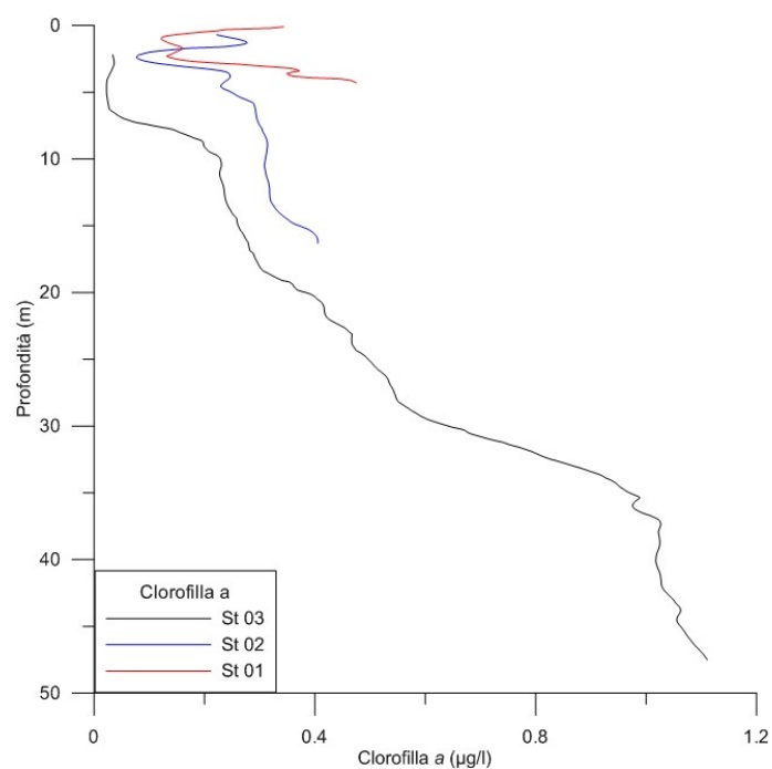
Fig. 9 Andamento della Clorofilla a nelle Stazioni ST01PT, ST02PT, ST03PT durante le campagne FPOA_1
