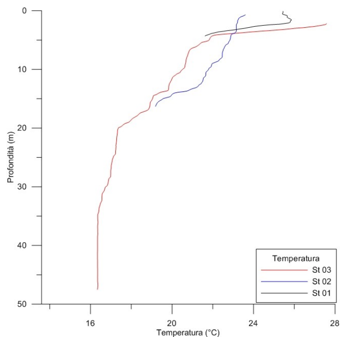
Fig. 4 Andamento della Temperatura nelle Stazioni ST01PT, ST02PT, ST03PT durante le campagne FPOA_1
