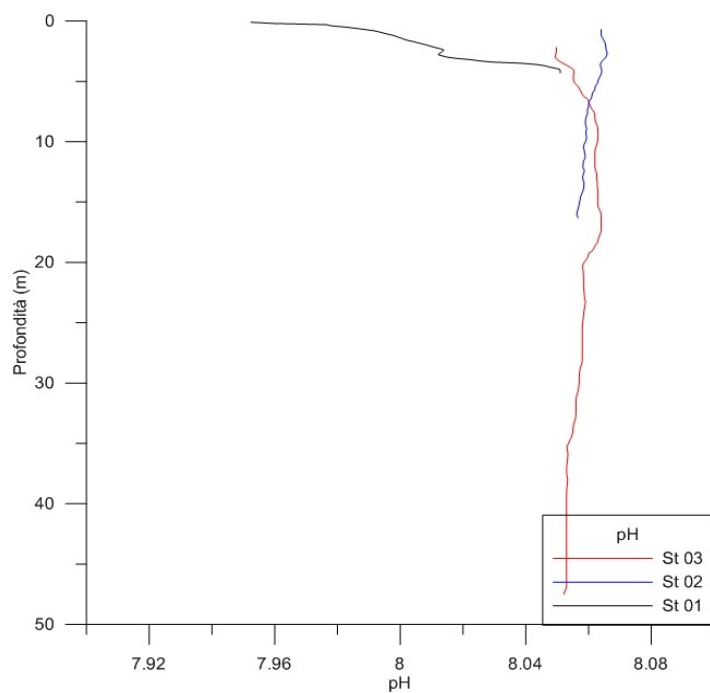
Fig. 7 Andamento della pH nelle Stazioni ST01PT, ST02PT, ST03PT durante le campagne FPOA_1
