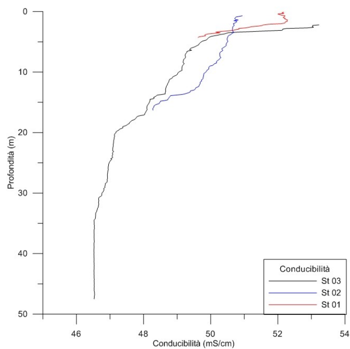
Fig. 5 Andamento della Conducibilità nelle Stazioni ST01PT, ST02PT, ST03PT durante le campagne FPOA_1
