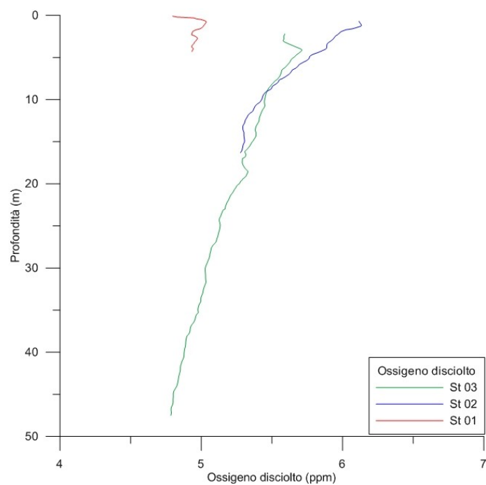
Fig. 8 Andamento dell'Ossigeno disciolto nelle Stazioni ST01PT, ST02PT, ST03PT durante le campagne FPOA_1
