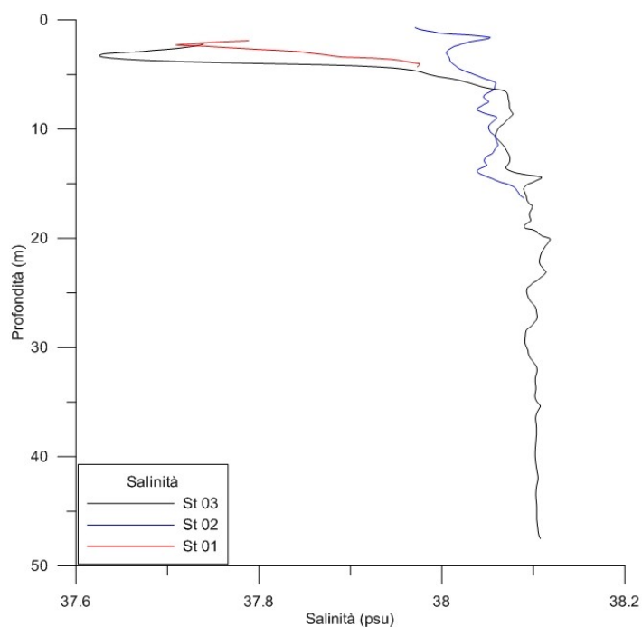
Fig. 6 Andamento della Salinità nelle Stazioni ST01PT, ST02PT, ST03PT durante le campagne FPOA_1
